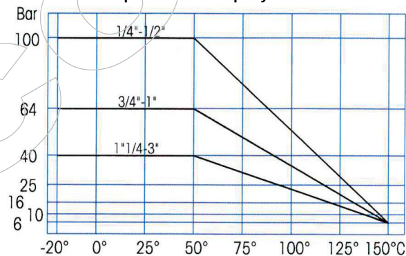
Graf závislosti provozního a teploty
