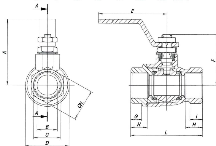
Tabulka rozměrů
